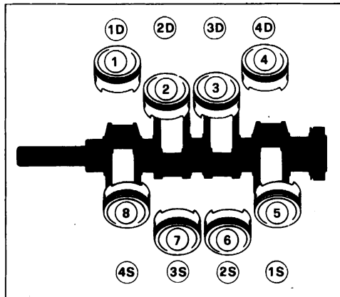
63) Pistons disposition.
