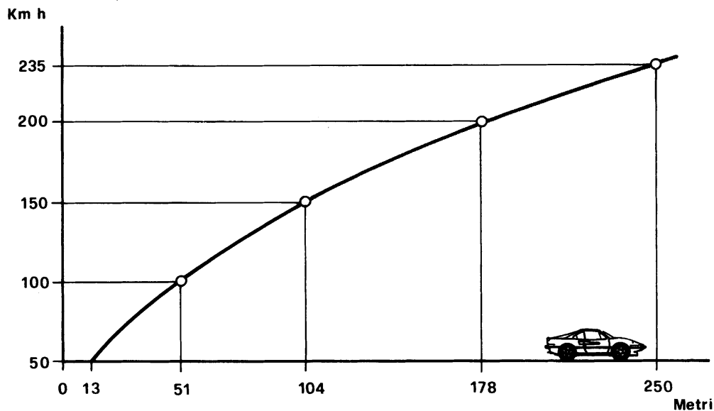
82) Diagramma spazio frenatura.
