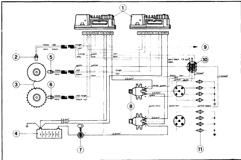
62) Ignition circuit layout.
