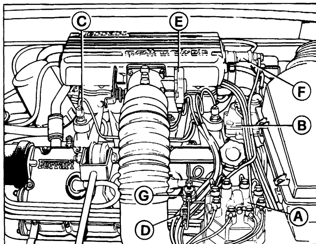
60) Injection system.
